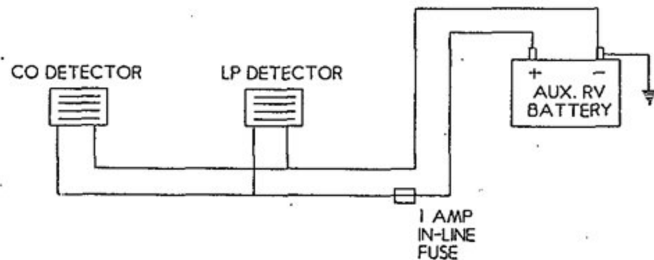
CO & LP DETECTOR WIRING
