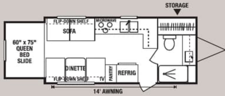
21JQ • UVW 4286 • Dry Hitch Wt. 510 • NCC 2714 • Length 22'4"
