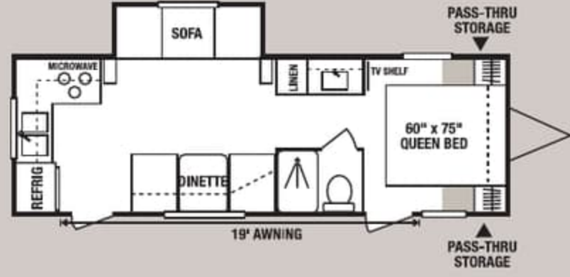
26JS • UVW 4870 • Dry Hitch Wt. 440 • NCC 2130 • Length 27'3"
