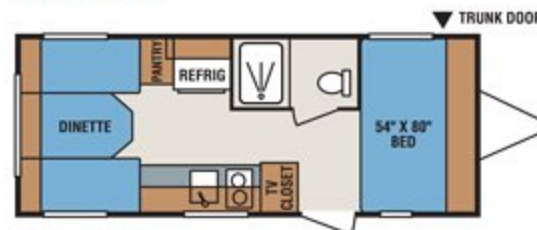
E19SB
