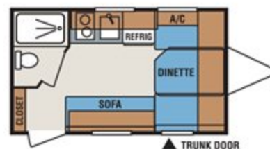
E14RB
