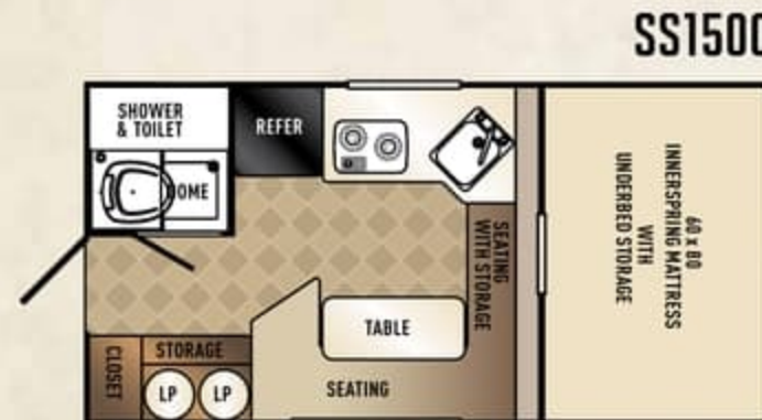
*CONÇU POUR CAMIONS PLEINE GRANDEUR AVEC 8' DE PLATEAU
