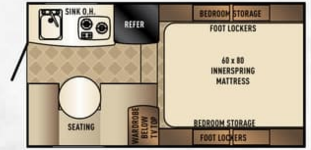
1/2 TON 5'6" OR 6'6" BED
