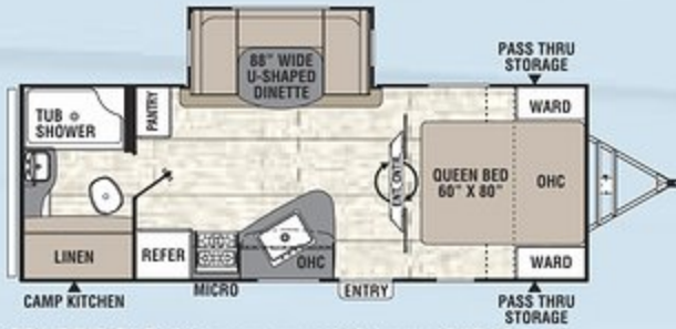
231 RBSLE / Longueur extérieure 26' 10"
