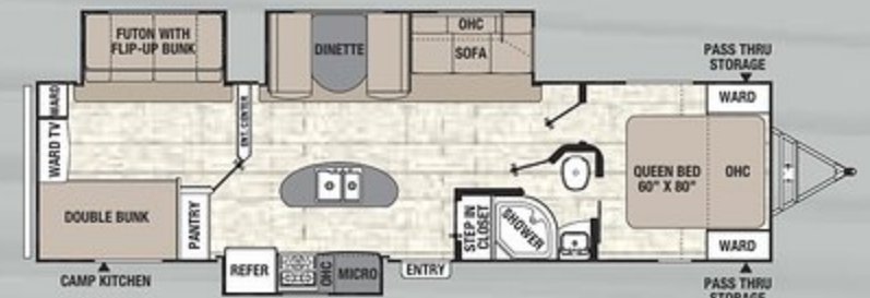
320 BHDS / Longueur extérieure 36' 11"
