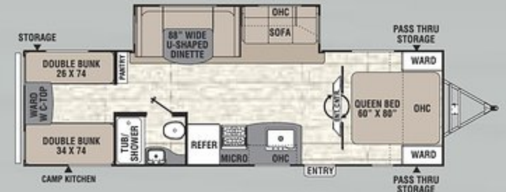
292 BHDS / Longueur extérieure 33' 5"
